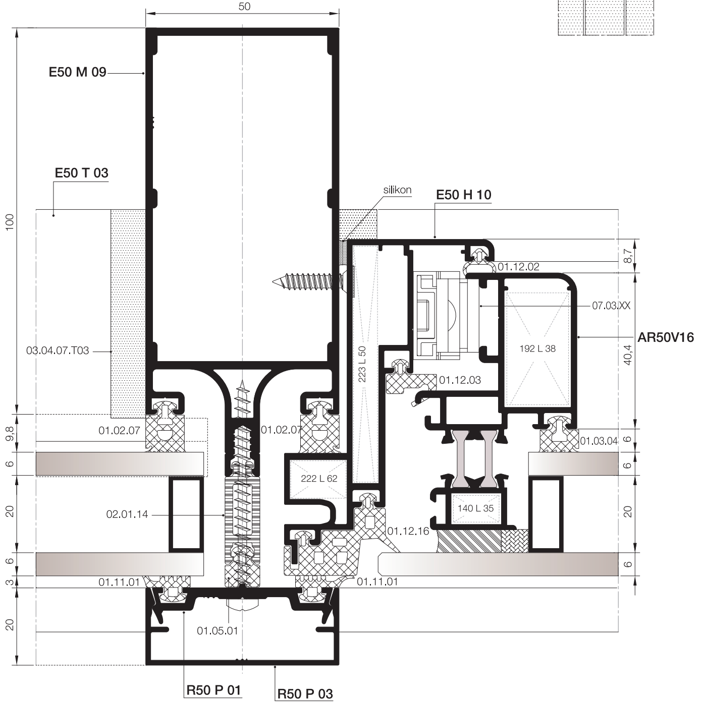
YATAY SİLİKON DÜŞEY KAPAKLI SİSTEM GİZLİ KANAT DÜŞEY DETAYI SEMI STRUCTURAL SYSTEM HIDDEN VENT VERTICAL DETAIL
